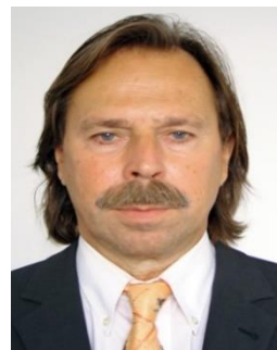
Hans Joachim Schmoll 2006
